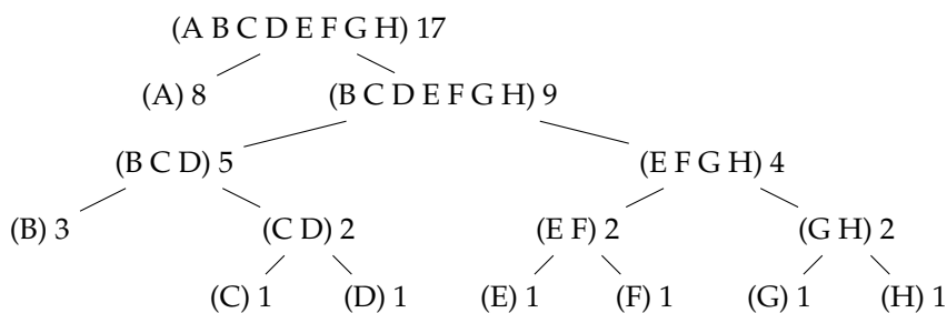
FIG. 1 – Un codage de Huffman encodé comme un arbre
